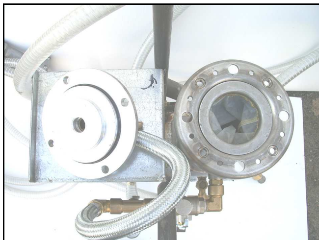
Vue sur le couvercle démontable et le filtre lavable
